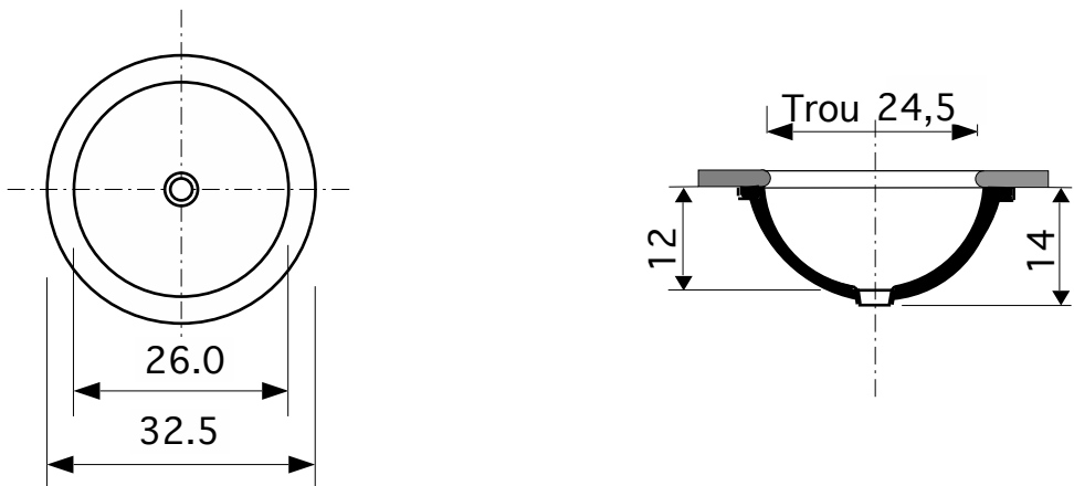
Vasque SANIBEL Ø26 en composite TRONYX
